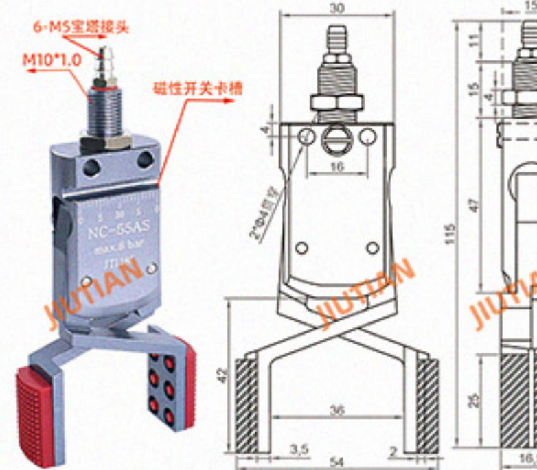
Mini-NC-55AS 夹取范围 54-78mm
