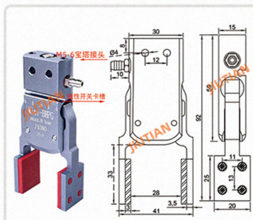
Mini-BHPG-25# 夹取范围 0-27MM
