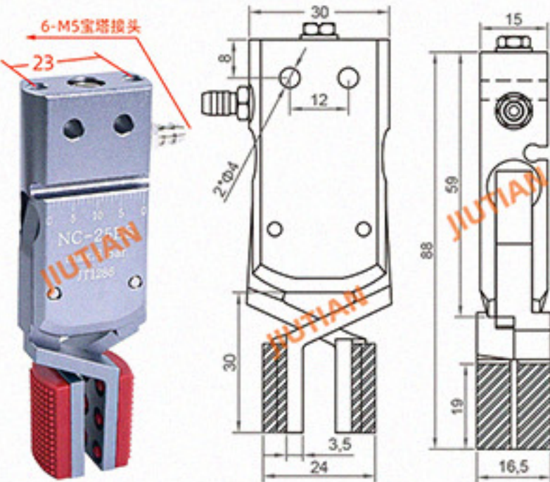
Mini-NC-25BS 夹取范围 24-42mm
