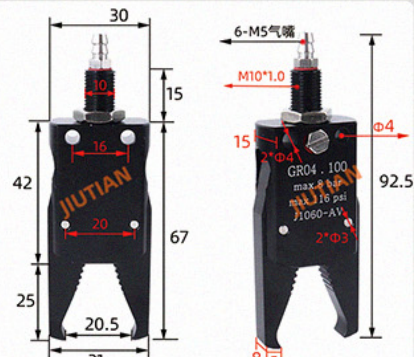
Mini-AV 外牙 夹取范围 0-20mm
