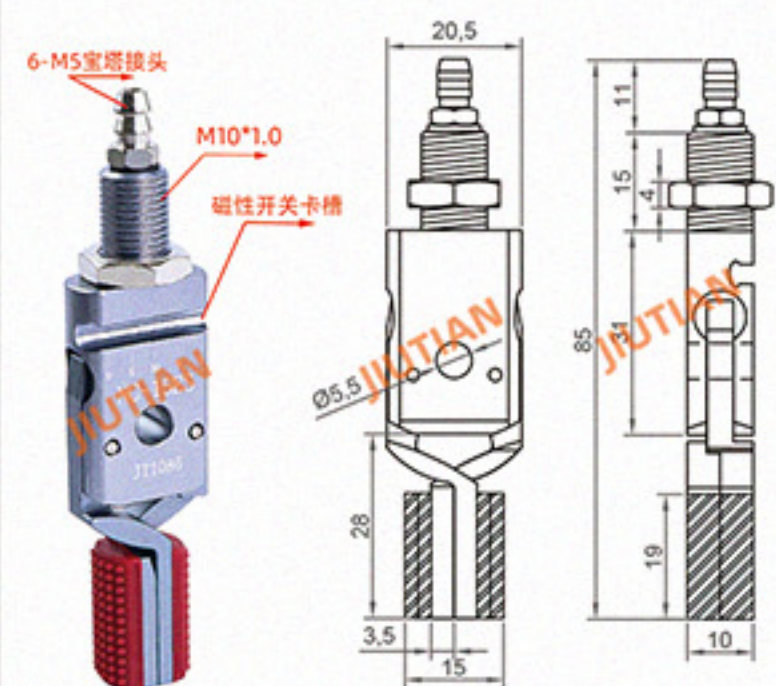
Mini-NC-15ES 夹取范围 15-30mm
