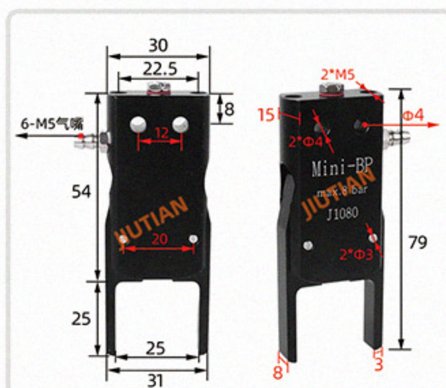
Mini-BP 夹取范围 5-25mm
