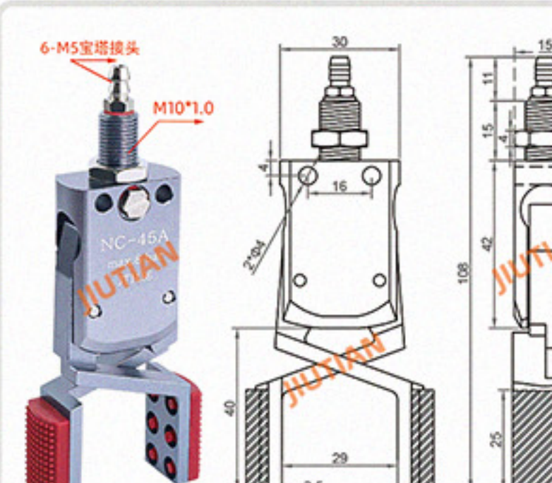
Mini-NC-45A 夹取范围 34-58mm
