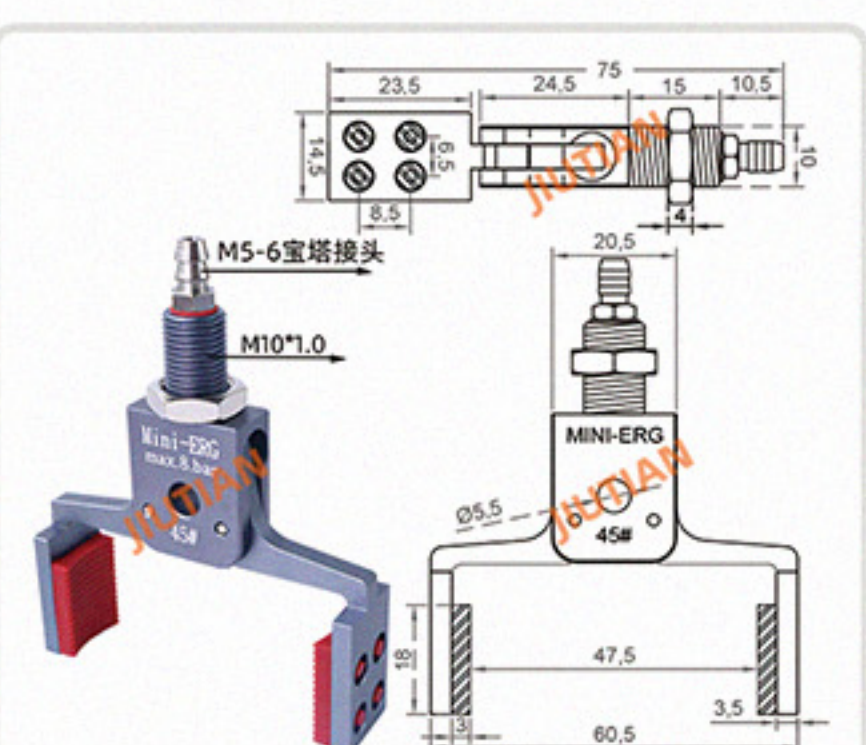
Mini-ERG-45# 夹取范围 31-47MM
