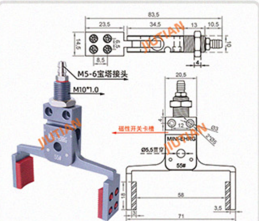
Mini-EHRG-55# 夹取范围 40-57MM
