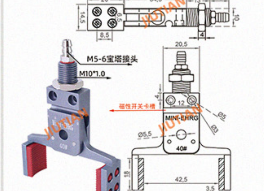
Mini-EHRG-40# 夹取范围 29-42MM
