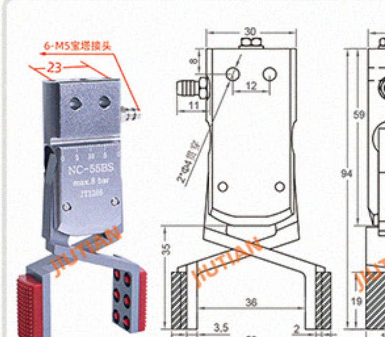
Mini-NC-45BS 夹取范围 54-78mm
