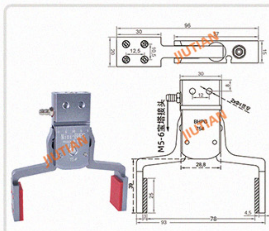
Mini-BHPG-75# 夹取范围 42-78MM
