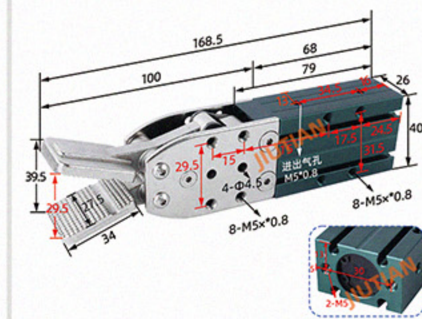
单动 (接 1 根气管) 2015S
