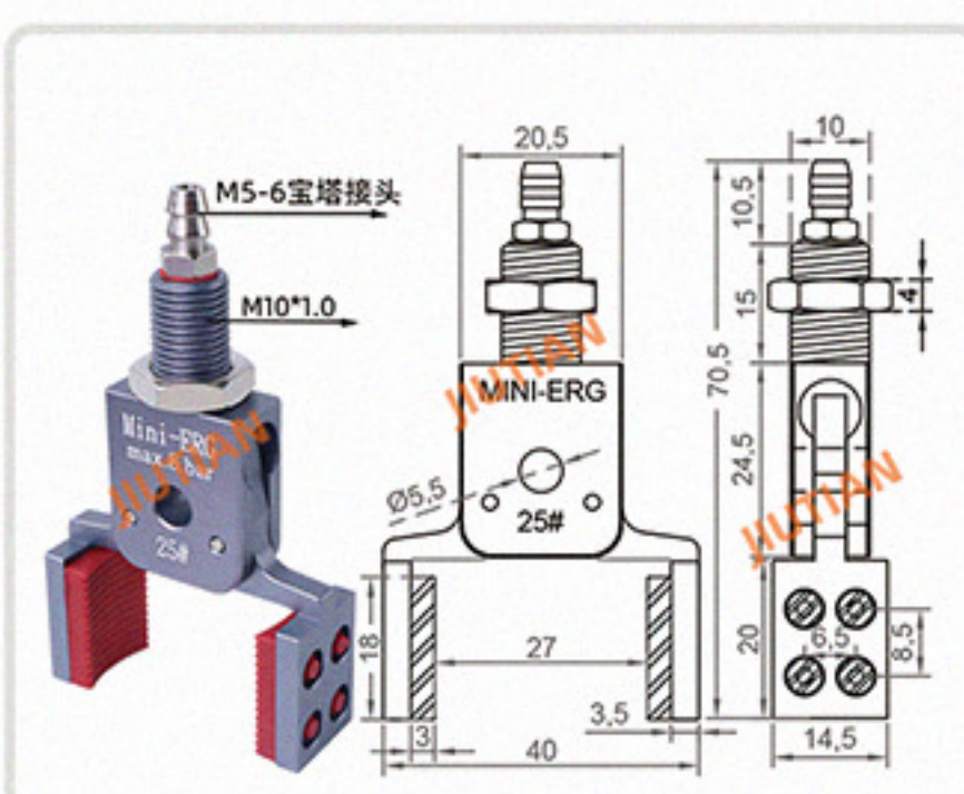
Mini-ERG-25# 夹取范围 15-26MM
