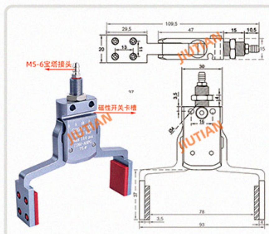
Mini-AHPG-75# 夹取范围 39-78MM
