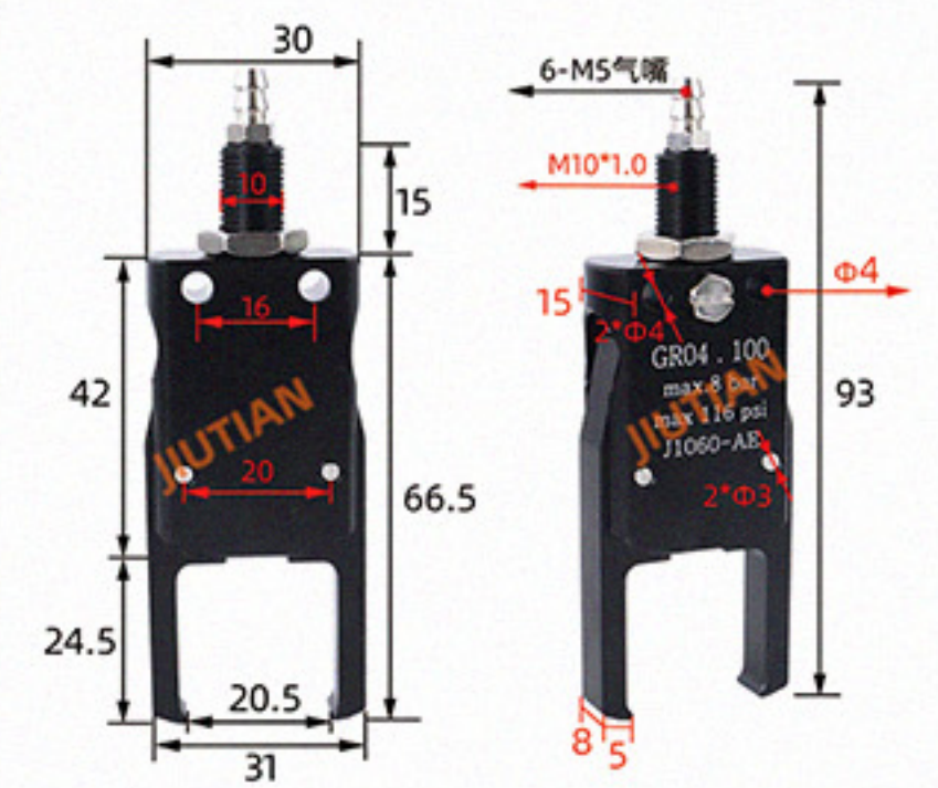
Mini-AE 外牙 夹取范围 0-20mm
