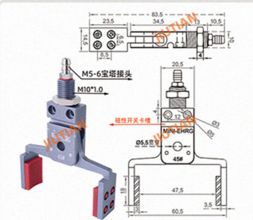
Mini-EHRG-45# 夹取范围 31-47MM
