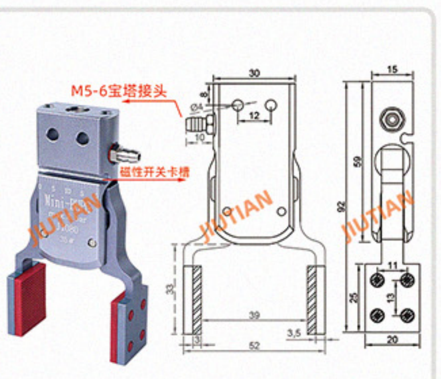
Mini-BHPG-35# 夹取范围 9-38MM
