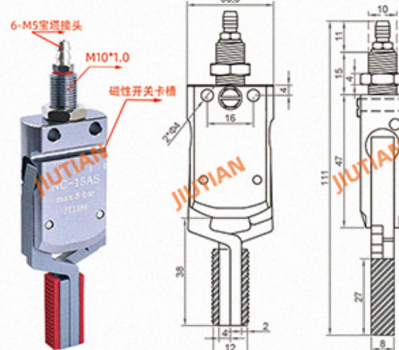
Mini-NC-15AS 夹取范围 13-33mm
