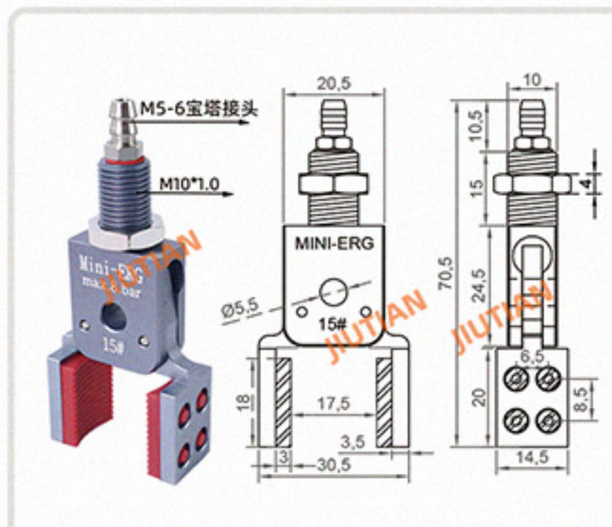
Mini-ERG-15# 夹取范围 5-17MM
