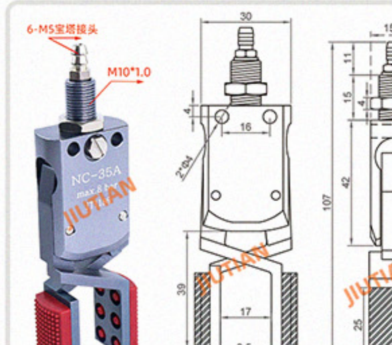
Mini-NC-35A 夹取范围 23-45mm
