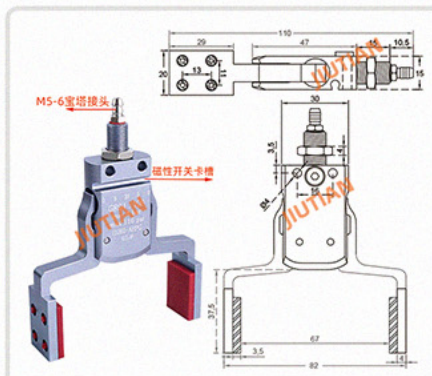
Mini-AHPG-65# 夹取范围 33-66MM
