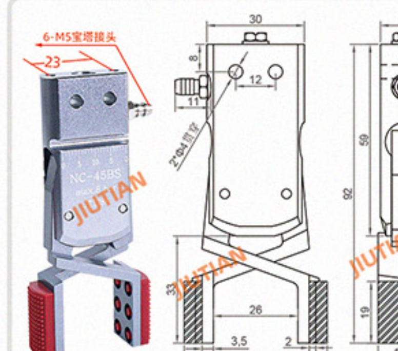
Mini-NC-45BS 夹取范围 44-66mm
