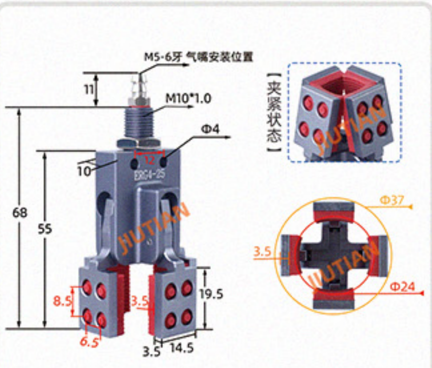
ERG-4-25# 夹取范围 10-24MM
