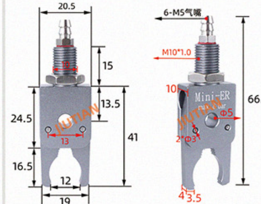
Mini-ER 顶进气 夹取范围 4-12MM
