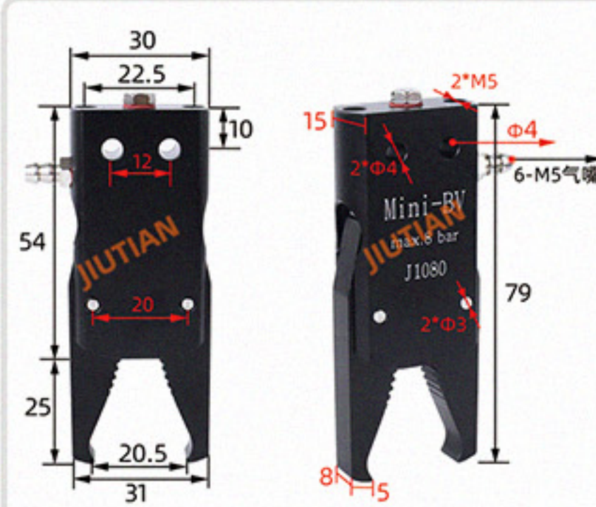
Mini-BV 侧进气 夹取范围 0-20mm
