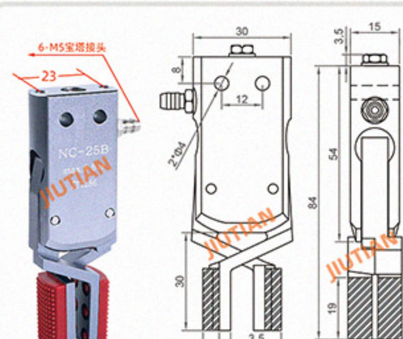
Mini-NC-25B 夹取范围 24-42mm
