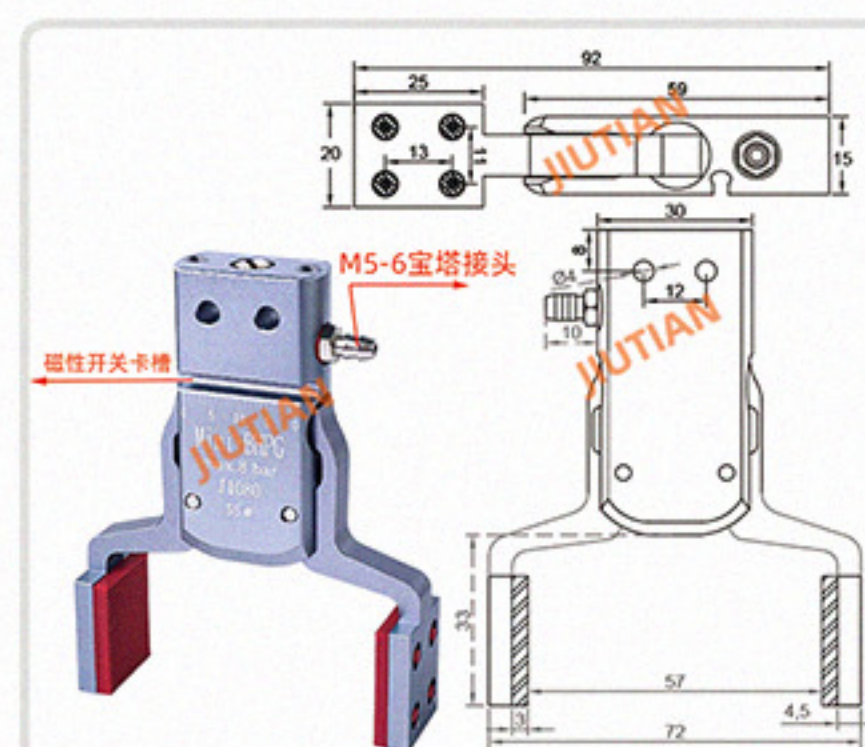
Mini-BHPG-55# 夹取范围 28-56MM
