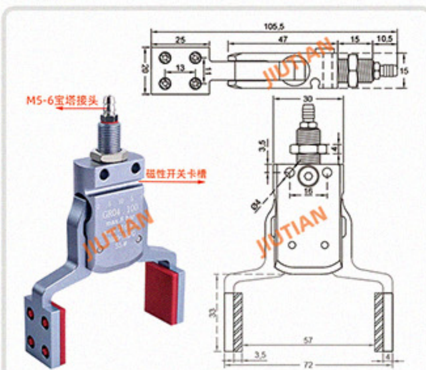
Mini-AHPG-55# 夹取范围 28-56MM
