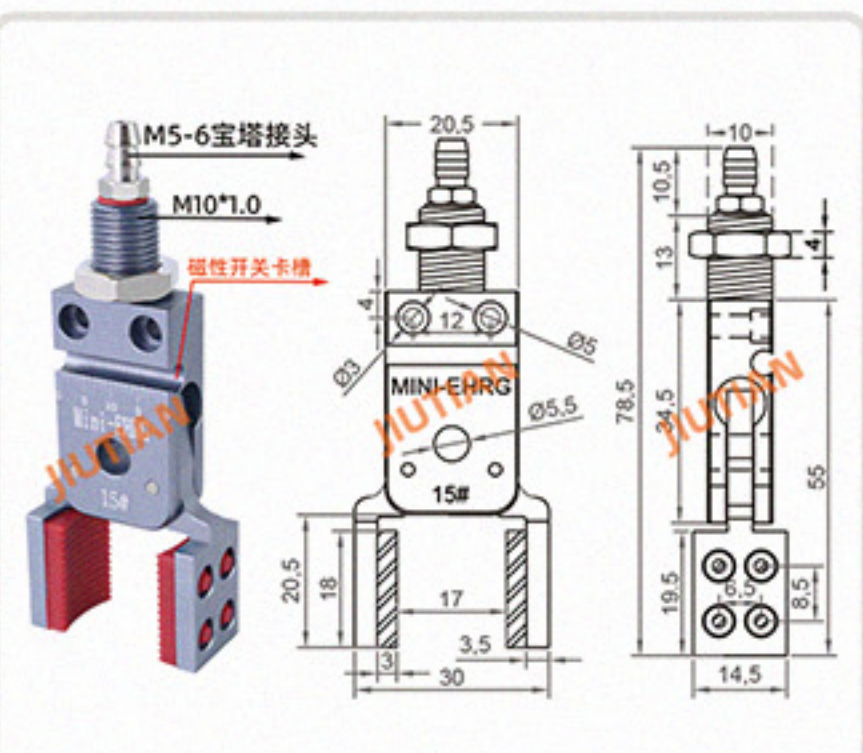
Mini-EHRG-15# 夹取范围 5-16MM
