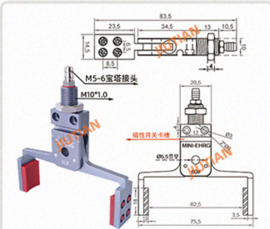
Mini-EHRG-60# 夹取范围 45-62MM
