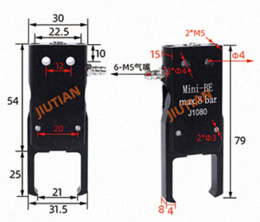
Mini-BE 侧进气 夹取范围 0-21mm
