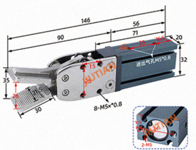
双动 ( 接 2 根气管 ) 1615D
