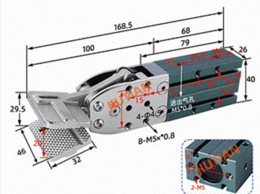
双动（加宽夹片）2015D-L
