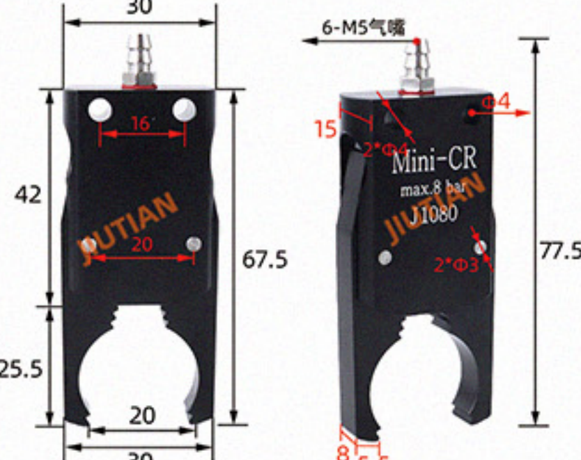
Mini-CR 顶进气 夹取范围 9-20MM
