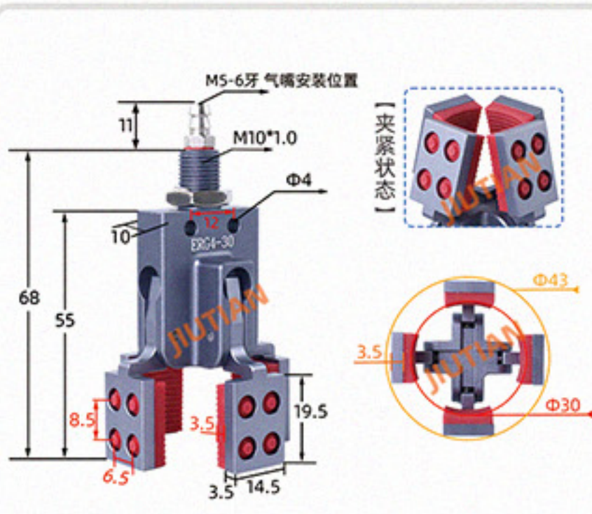
ERG-4-30# 夹取范围 14-30MM
