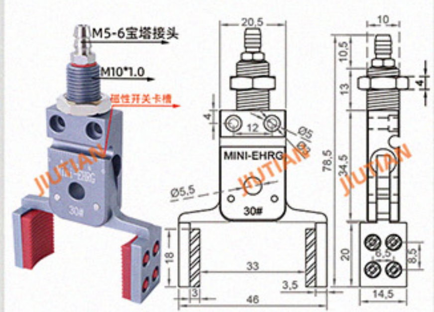
Mini-EHRG-30# 夹取范围 19-32MM
