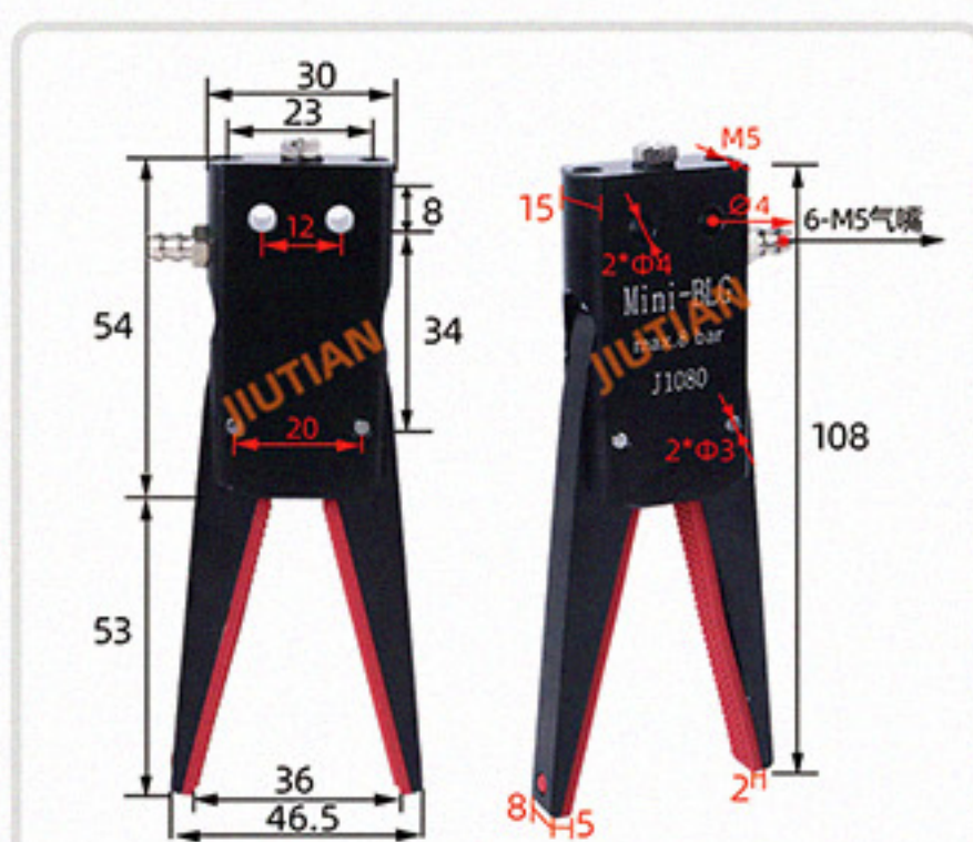
Mini-BLG侧进气 夹取范围 0-36mm
