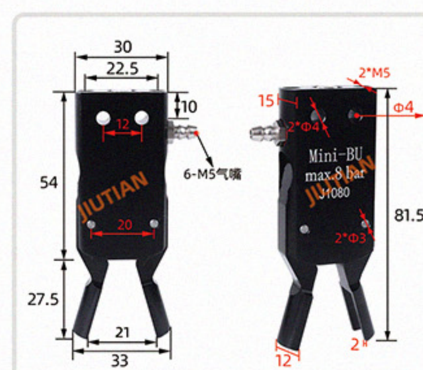
Mini-BU 侧进气 夹取范围 7-21mm
