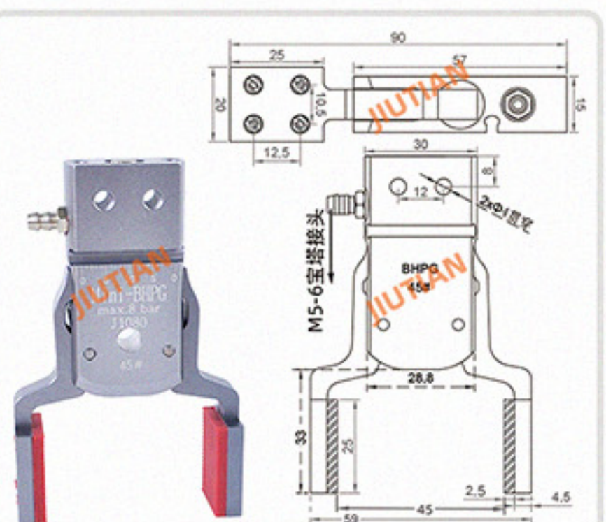
Mini-BHPG-45# 夹取范围 17-44MM
