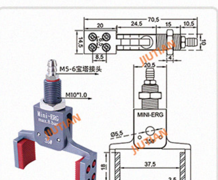
Mini-ERG-35# 夹取范围 24-37MM
