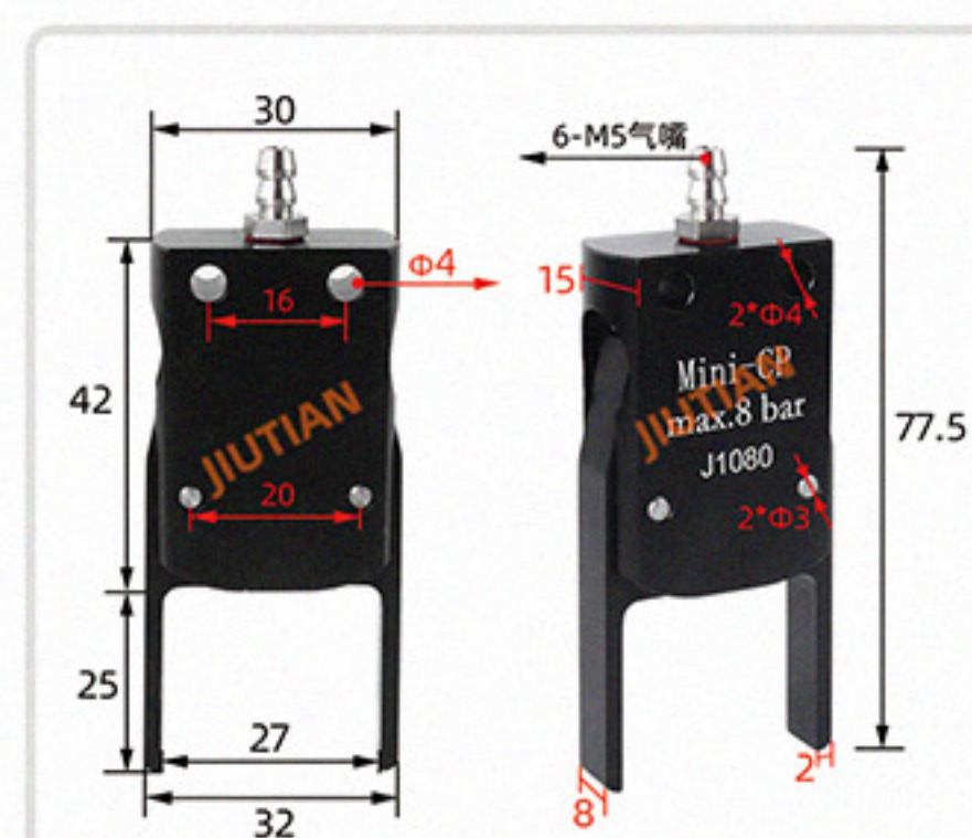
Mini-CP 夹取范围 5-25mm
