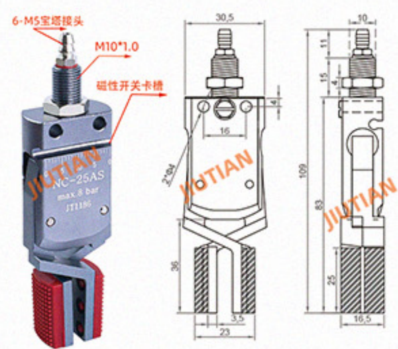
Mini-NC-25AS 夹取范围 25-46mm
