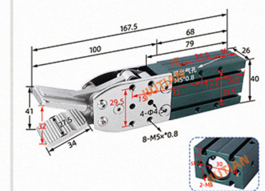
双动 (接 2 根气管) 2015D
