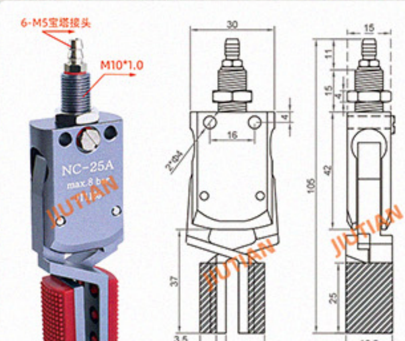
Mini-NC-25A 夹取范围 23-45mm
