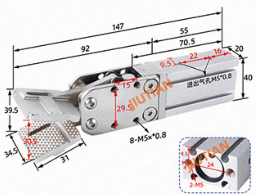
双动 (加宽夹片) 1615D-I
