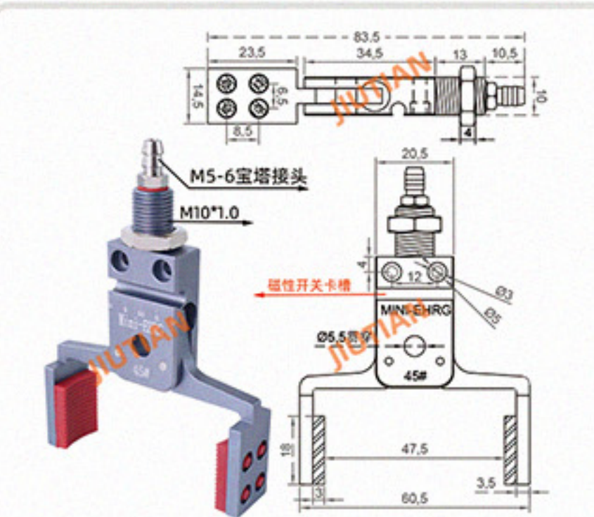
Mini-EHRG-45# 夹取范围 31-47MM
