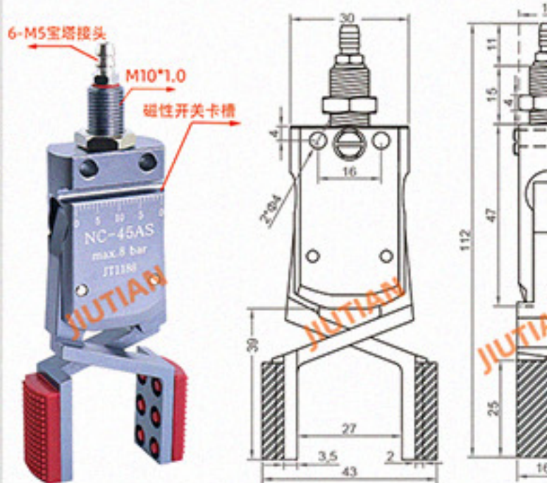
Mini-NC-45AS 夹取范围 45-66mm
