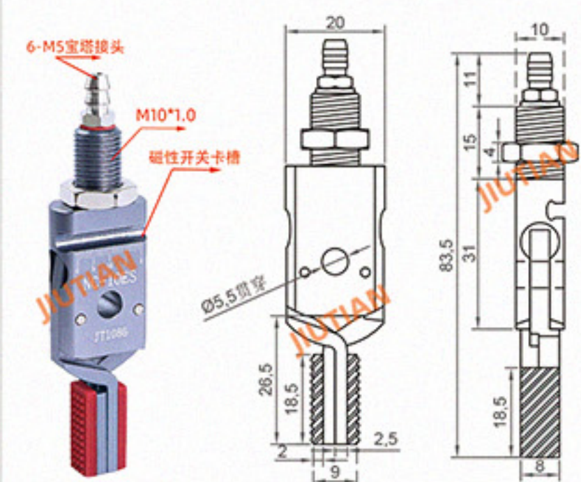
Mini-NC-10ES 夹取范围 10-26mm
