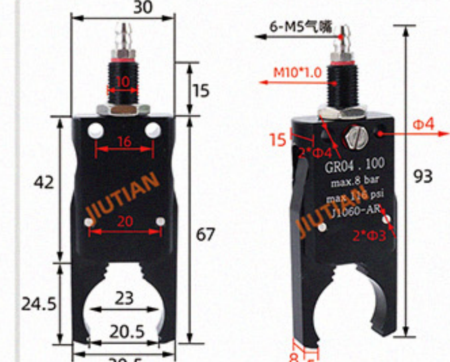
Mini-AR 外牙 夹取范围 9-20MM
