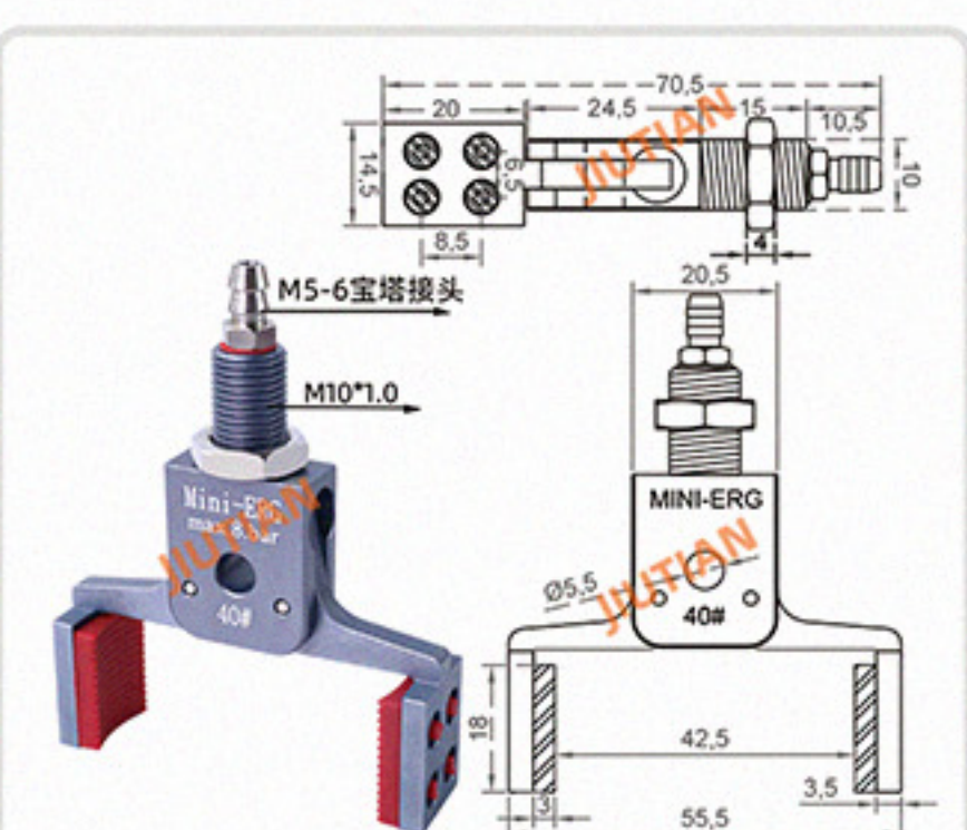
Mini-ERG-40# 夹取范围 29-42MM
