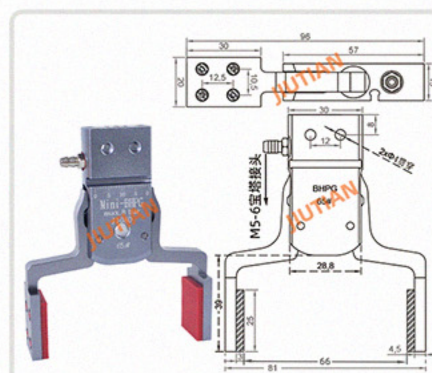
Mini-BHPG-65# 夹取范围 32-65MM
