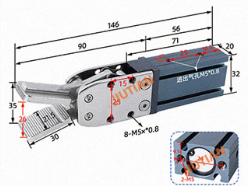
单动 (接 1 根气管) 1615S
