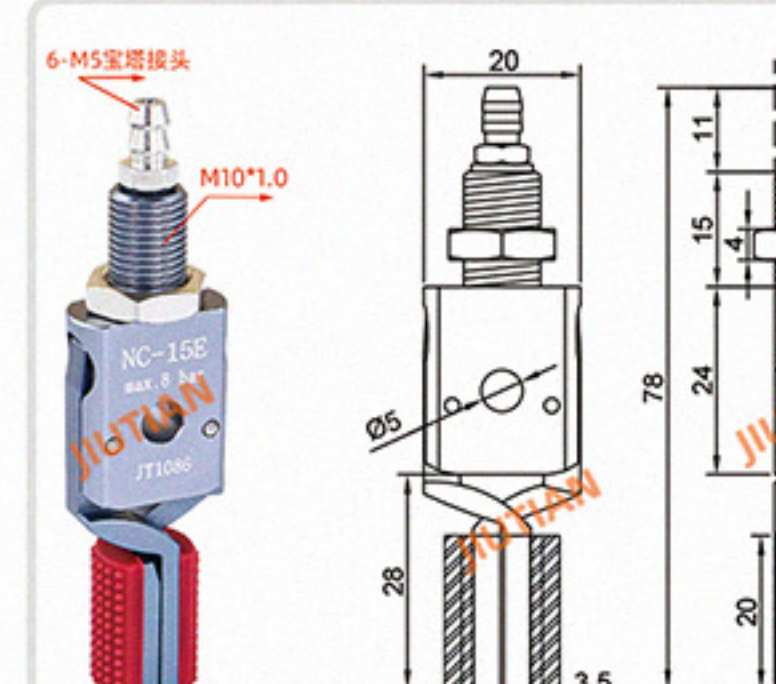
Mini-NC-15E 夹取范围 14-30mm
