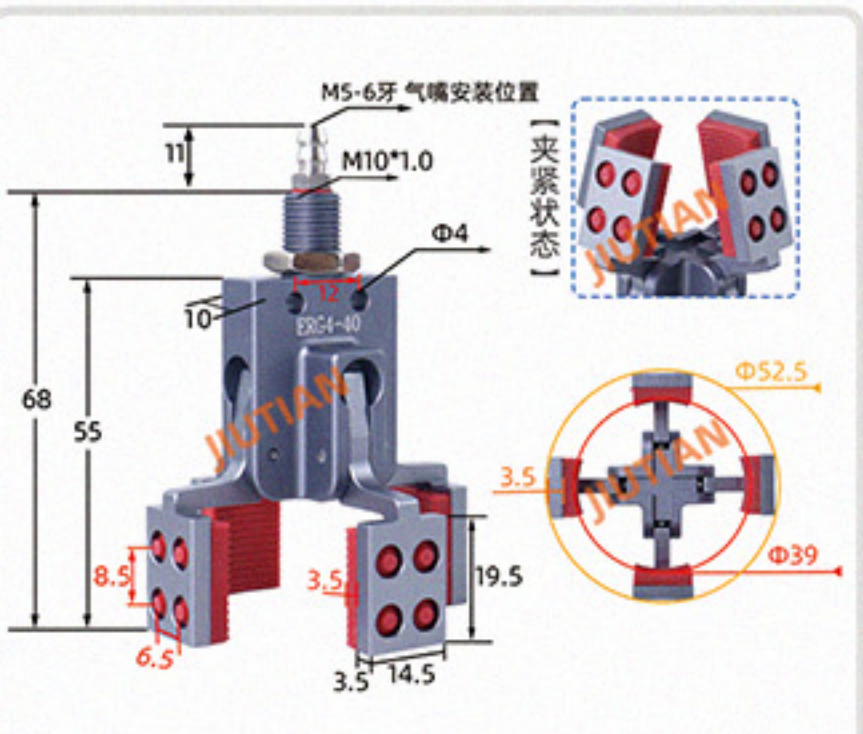
ERG-4-40# 夹取范围 25-39MM
