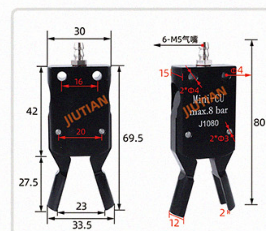
Mini-CU 顶进气 夹取范围 7-23mm
