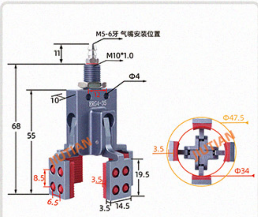
ERG-4-35# 夹取范围 19-34MM
