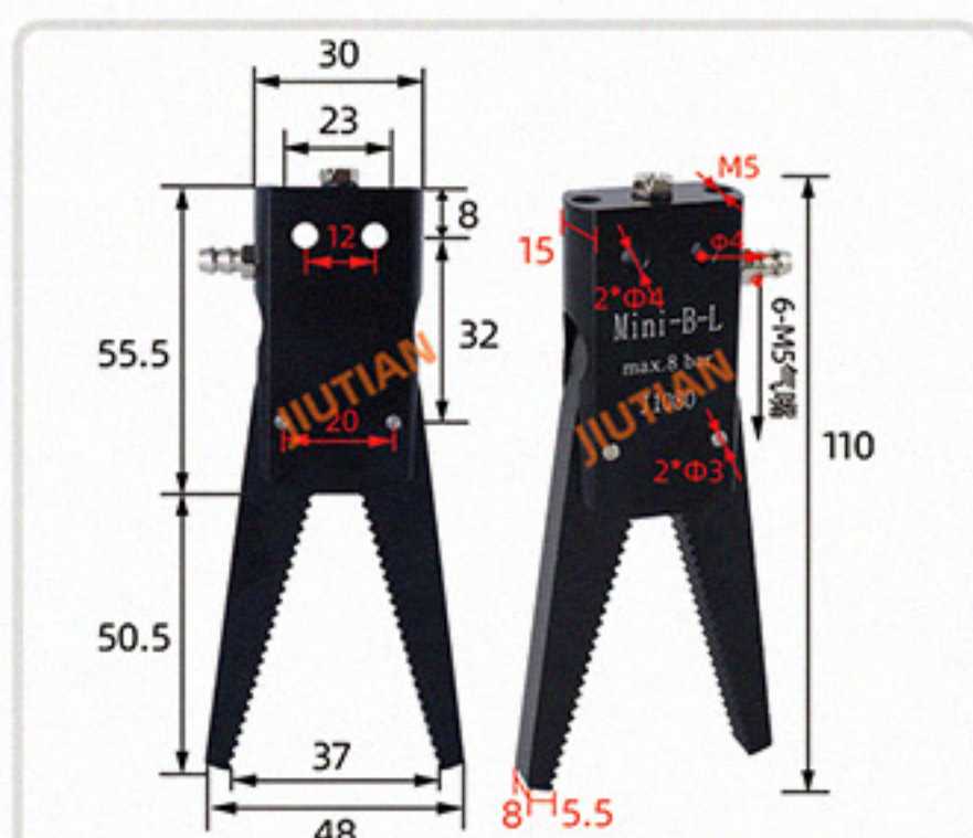
Mini-B-L侧进气 夹取范围 0-37mm
