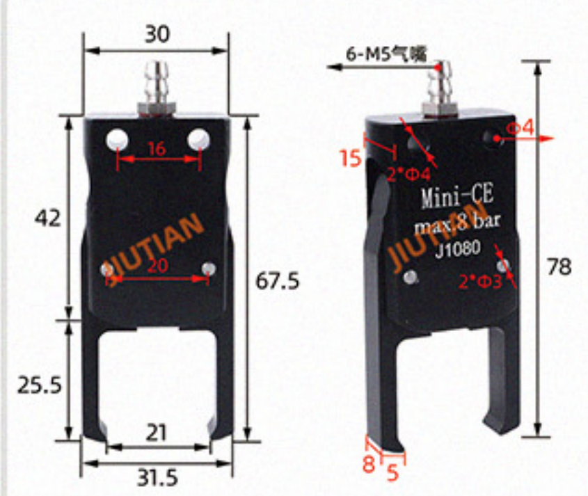
Mini-CE 顶进气 夹取范围 0-21mm
