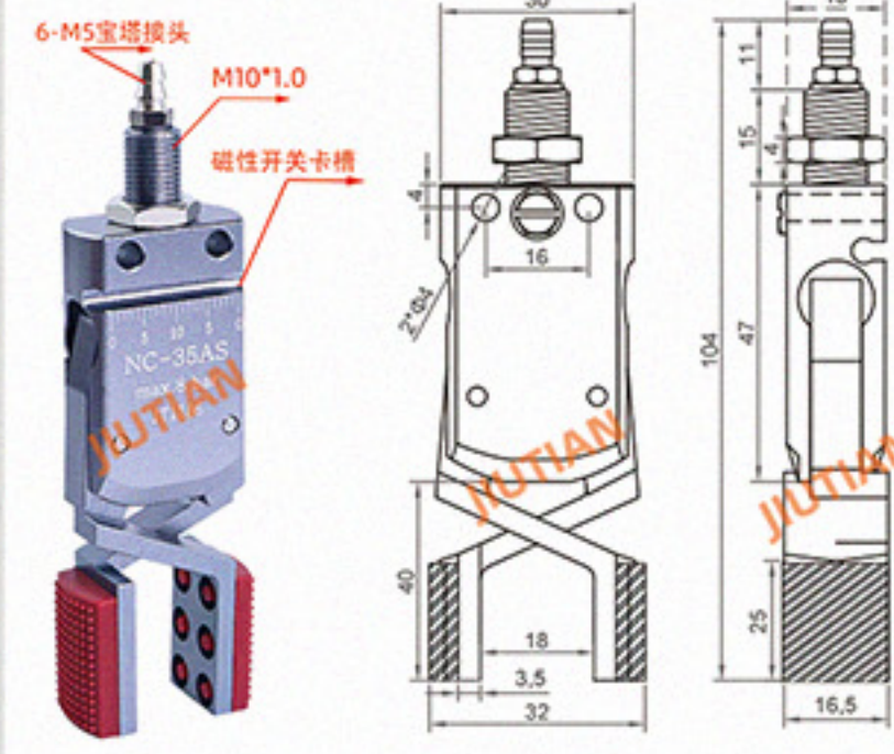
Mini-NC-35AS 夹取范围 34-60mm
