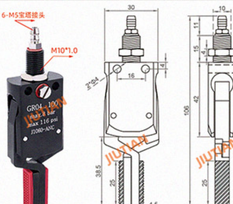
Mini-ANC 夹取范围 13-33mm
