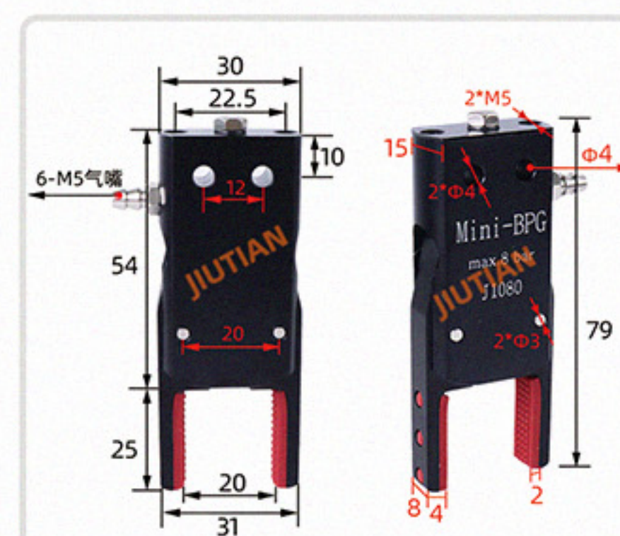
Mini-BPG 夹取范围 0-20mm
