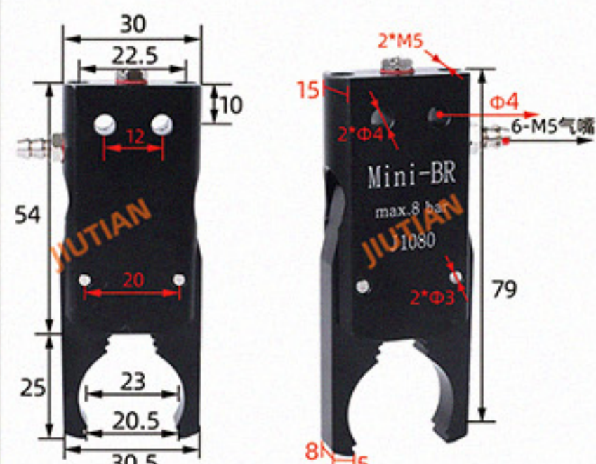
Mini-BR 侧进气 夹取范围 9-20MM
