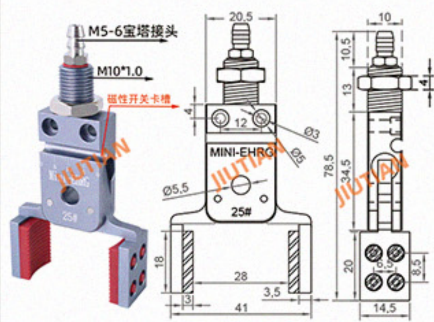
Mini-EHRG-25# 夹取范围 14-27MM
