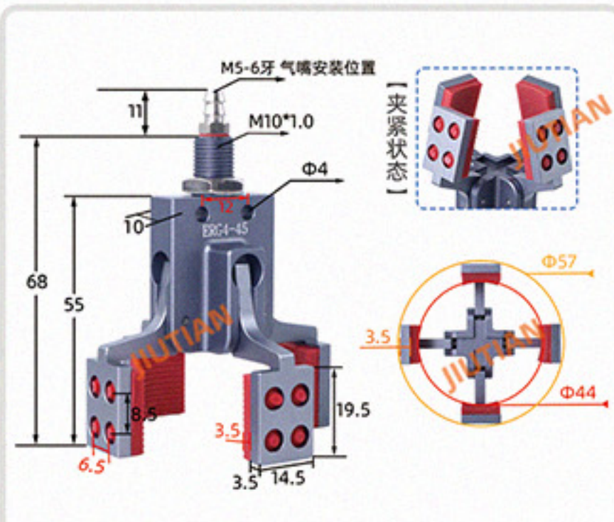
ERG-4-45# 夹取范围 30-44MM
