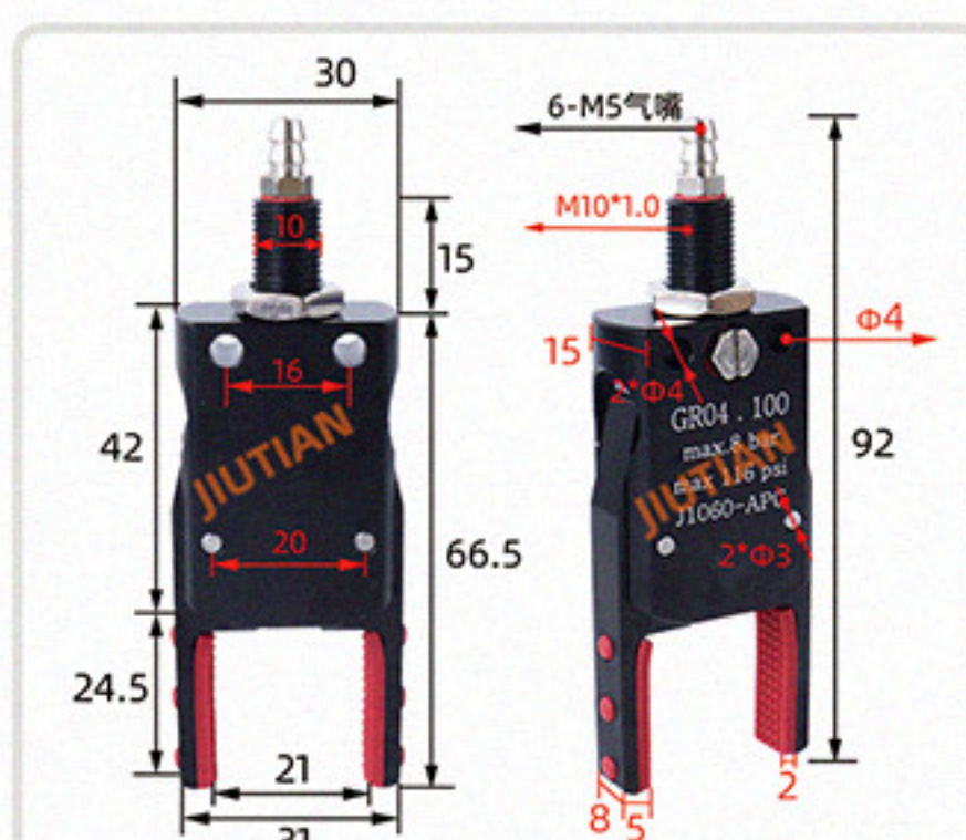
Mini-DPG 夹取范围 0-21mm
