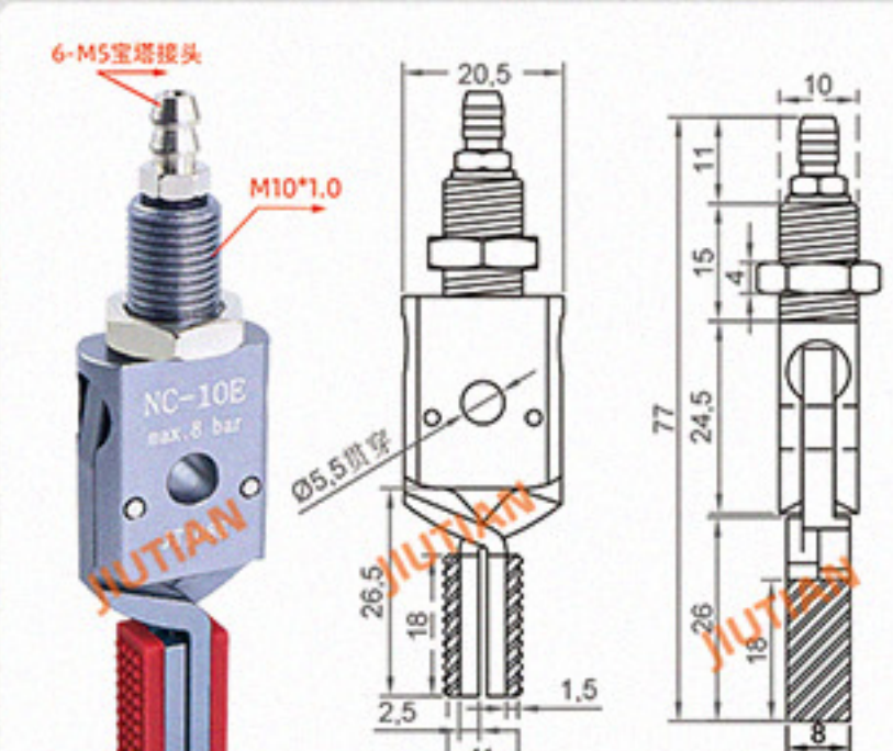
Mini-NC-10E 夹取范围 12-28mm
