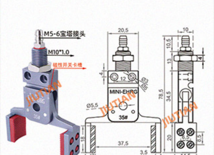
Mini-EHRG-35# 夹取范围 23-37MM
