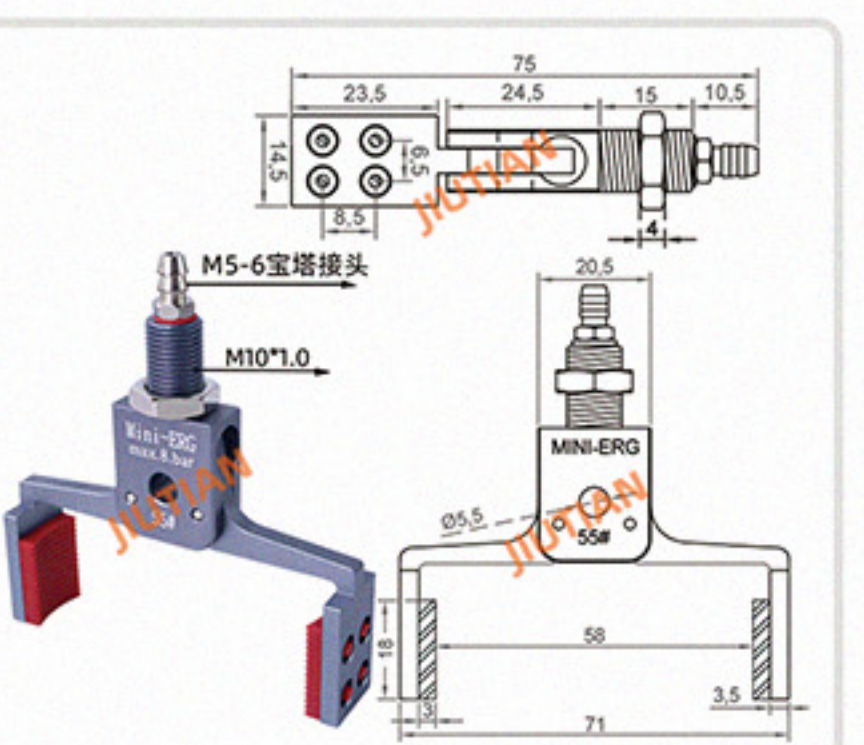
Mini-ERG-55# 夹取范围 41-57MM
