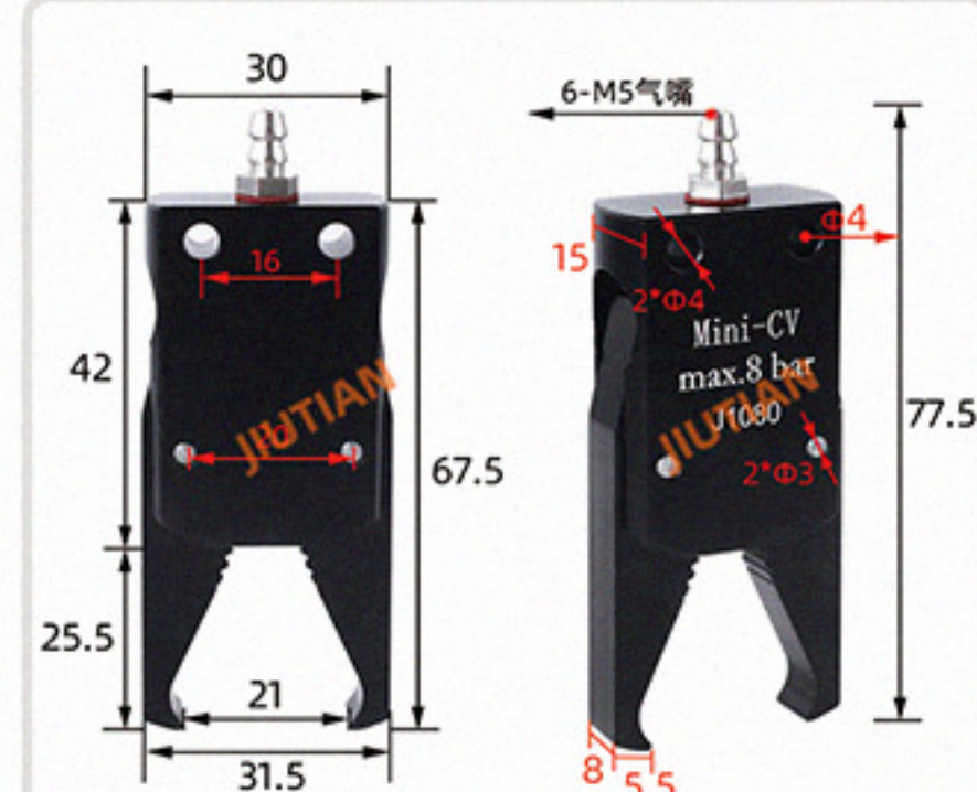
Mini-CV 顶进气 夹取范围 0-21mm
