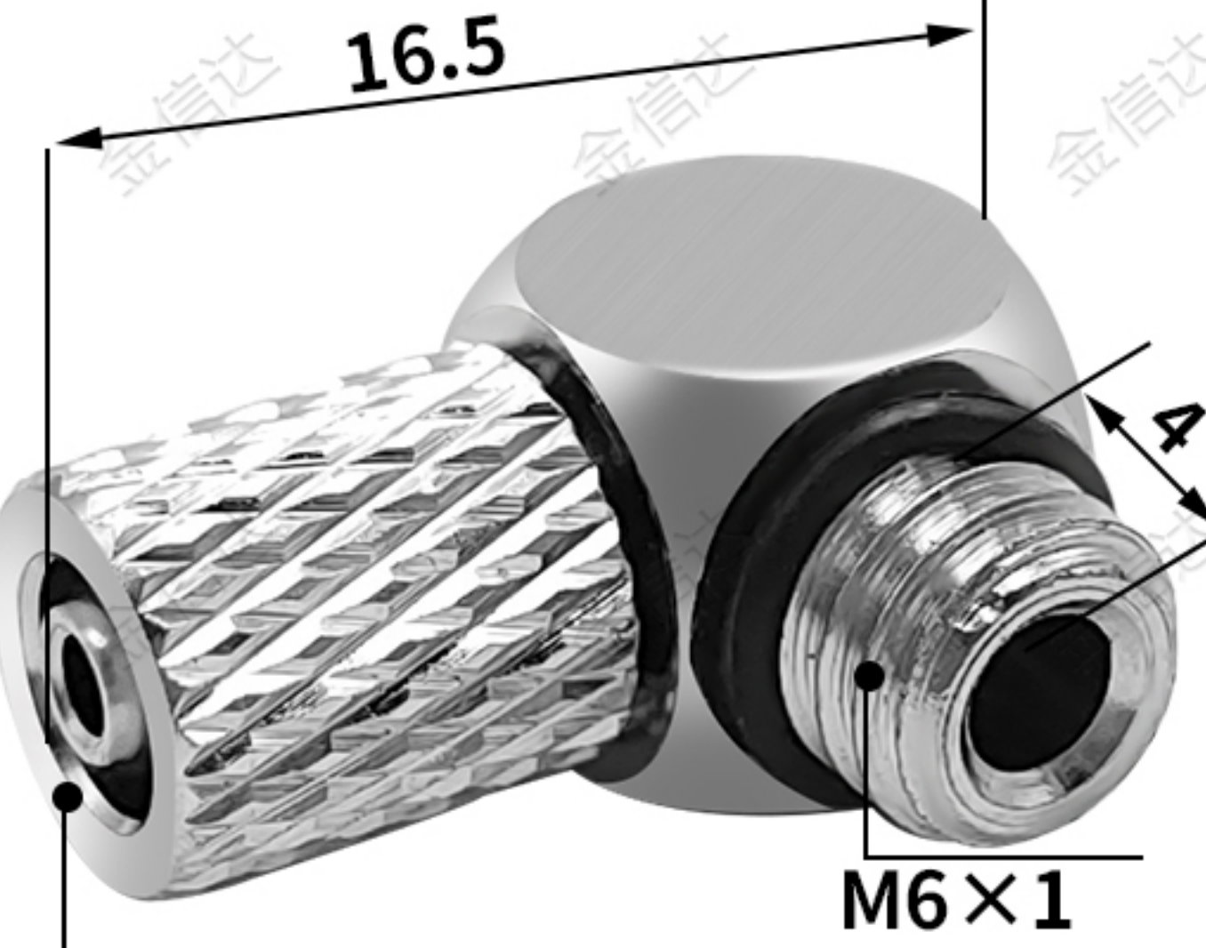
适配接管：4×2.5 Suitable Tube: 4×2.5
